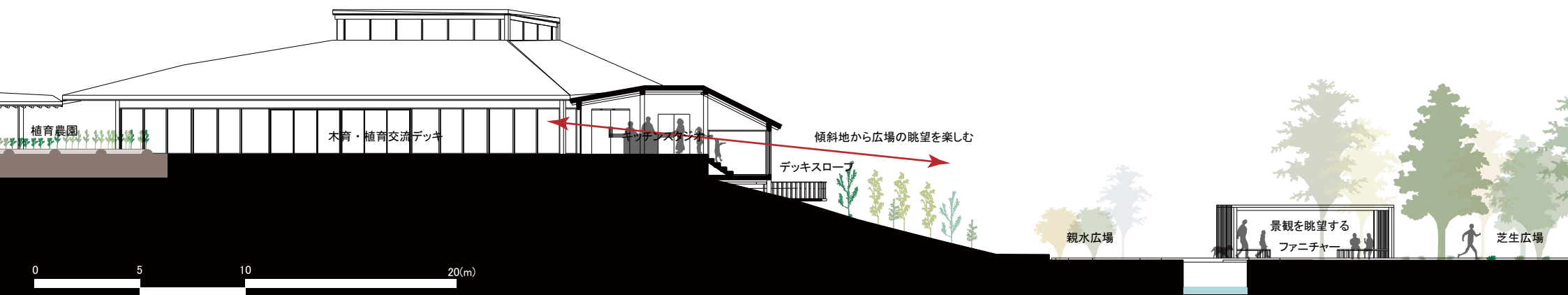
C-C' 断面図
